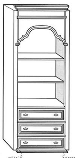
Art. 1517 Modulo Bizantino centrale 3 cass. + giorno Central element 3 drawers + open compart. Угловой Элемент 88x45x226 m 3 0,89
