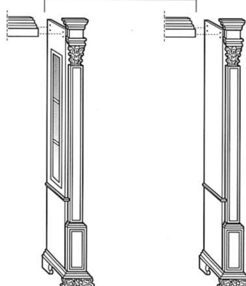
Art. 1532 Modulo Bizantino vetro gancio ponte dx-sx Element glass, hook, benches, dx-sx Угловой Элемент 15x45x226 m 3 0,15
